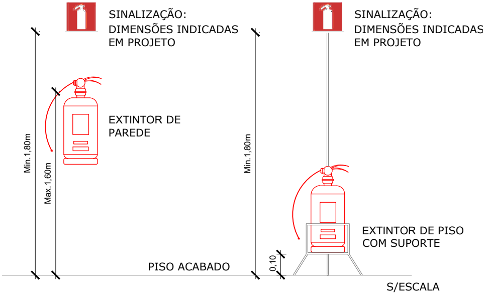
DETALHE DA FIXAÇÃO DO EXTINTOR DE INCÊNDIO
