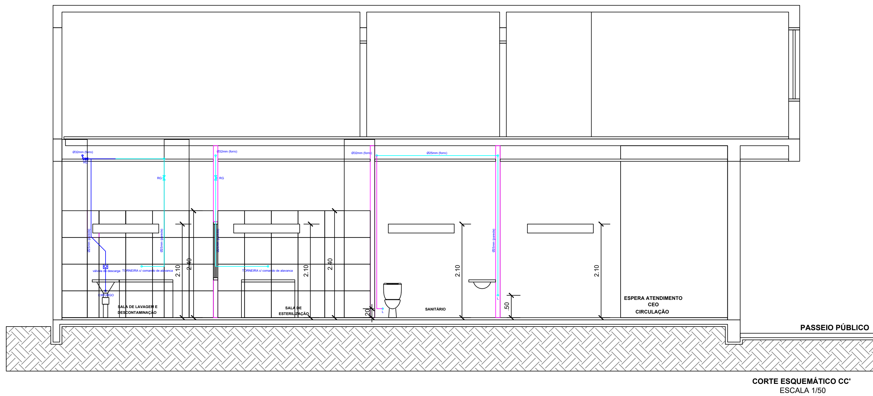
CORTE ESQUEMÁTICO CC' ESCALA 1/50
