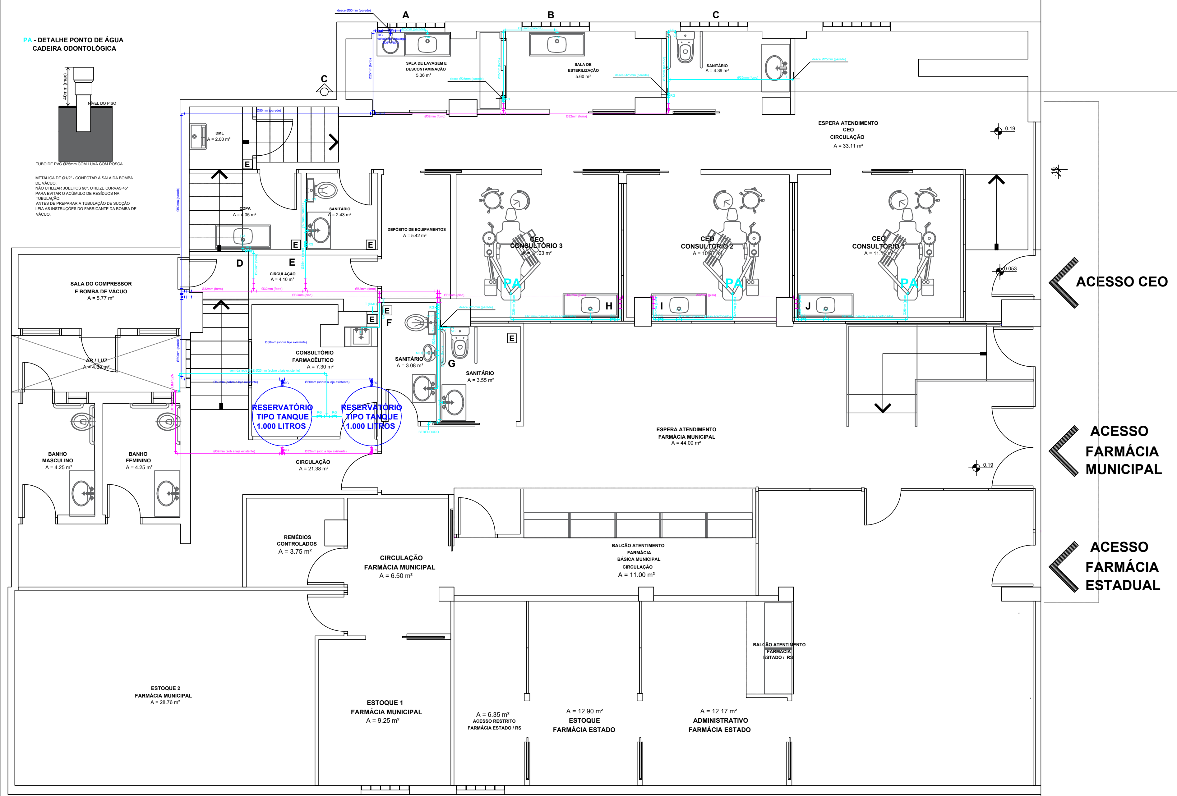
PLANTA BAIXA TÉRREO - REDE HIDRÁULICA ÁREA - 353,35 m² ESCALA 1/50
