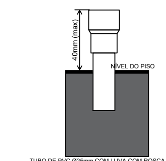
PA - DETALHE PONTO DE ÁGUA CADEIRA ODONTOLÓGICA
