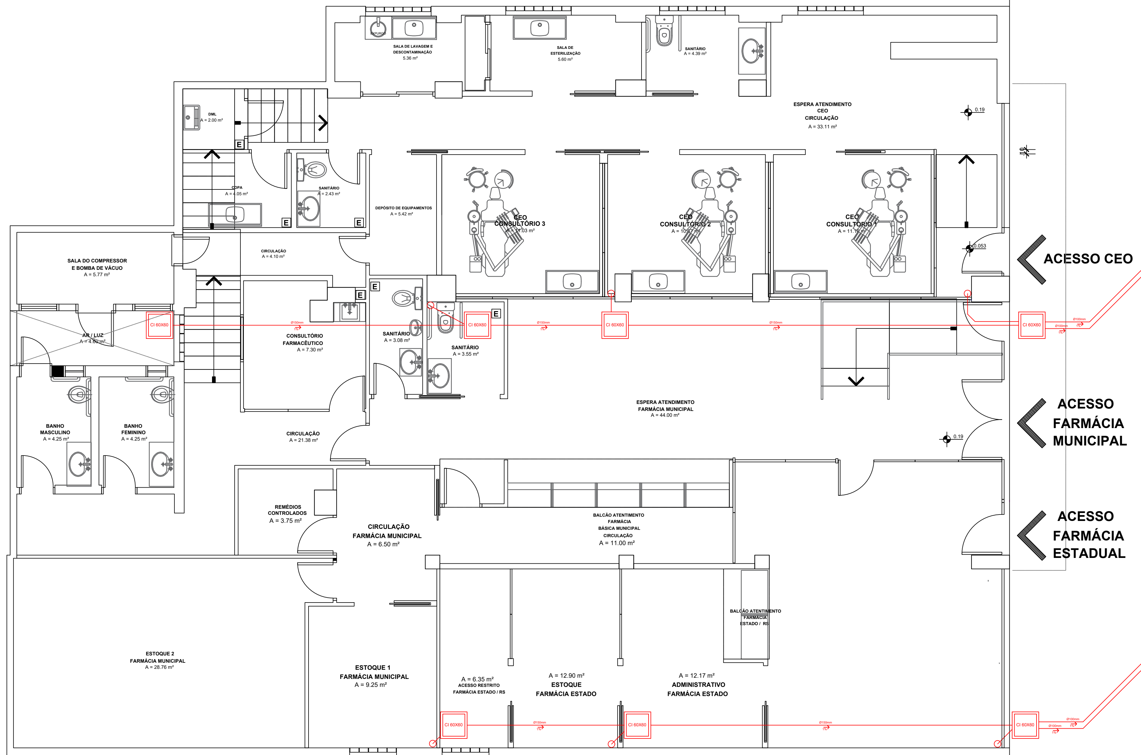
PLANTA BAIXA TÉRREO - REDE PLUVIAL ÁREA - 353.35 m² ESCALA 1/50
